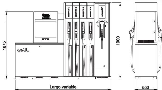
E30 A 84 GLP
