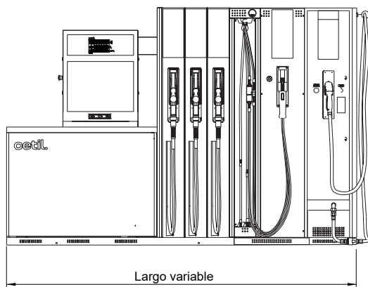
E30 A multiproducto con GNC
