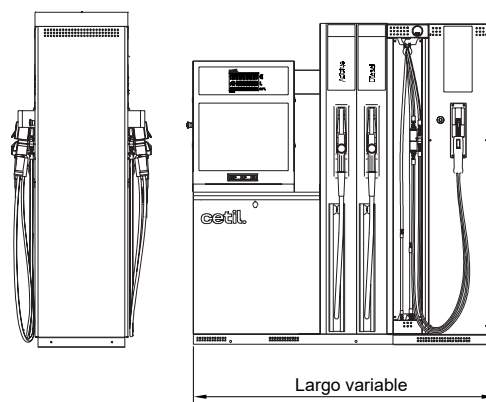
E30 A 42 con GNC
